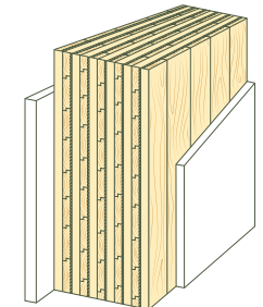
Obvodová stena – 11 vrstiev s vnútorným obložením a tenkou vonkajšou izoláciou
